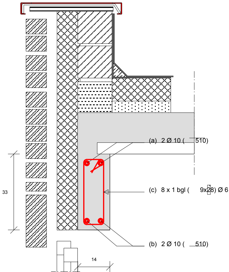
SNEDE A-A
