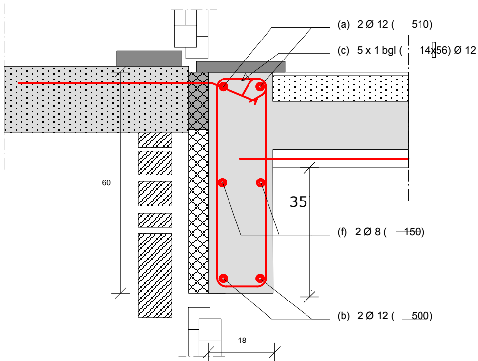
SNEDE A-A
