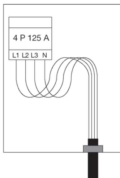
Aansluitkabel EXVB 4x10 - 4x16 - 4x25 mm 2
