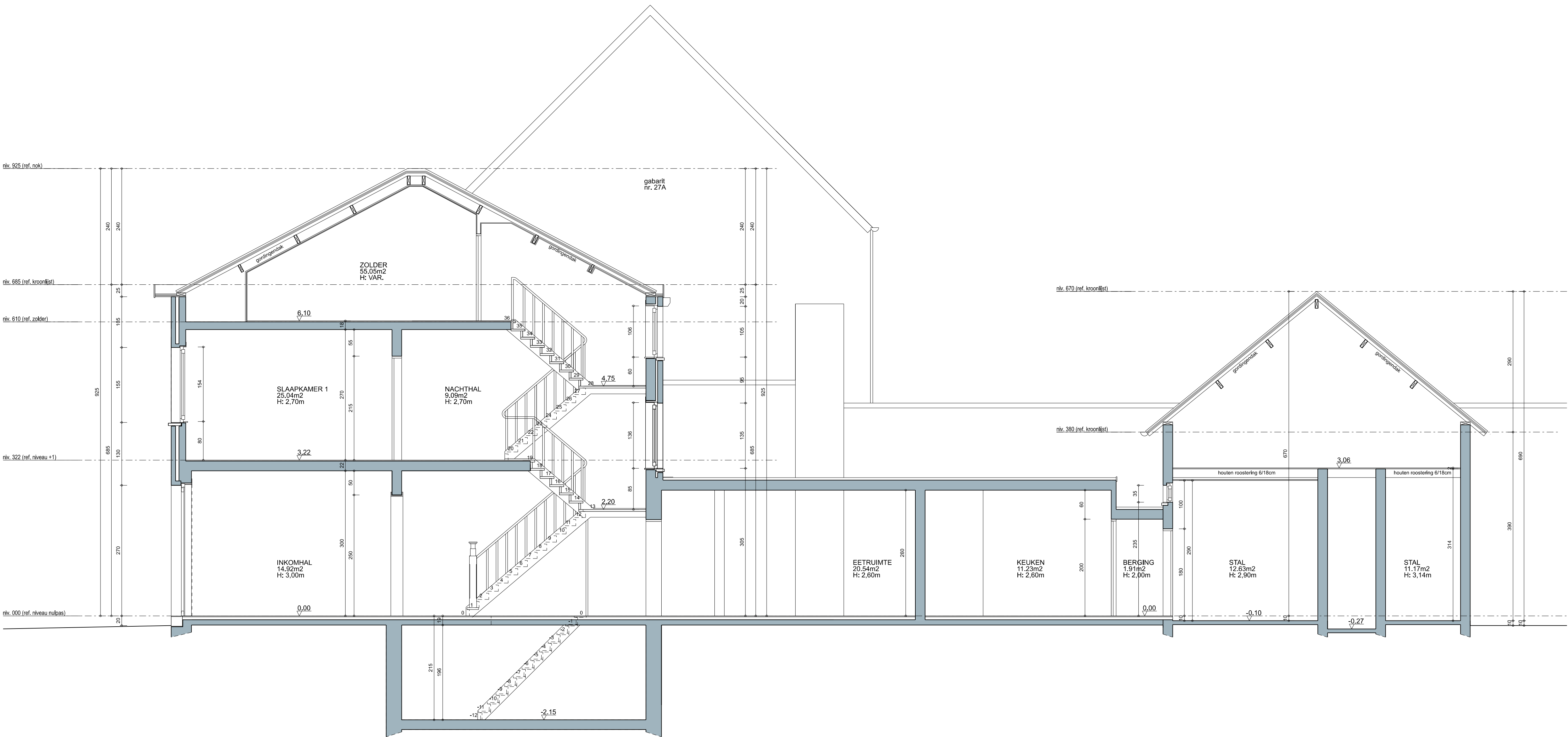
Doorsnede A-A'
