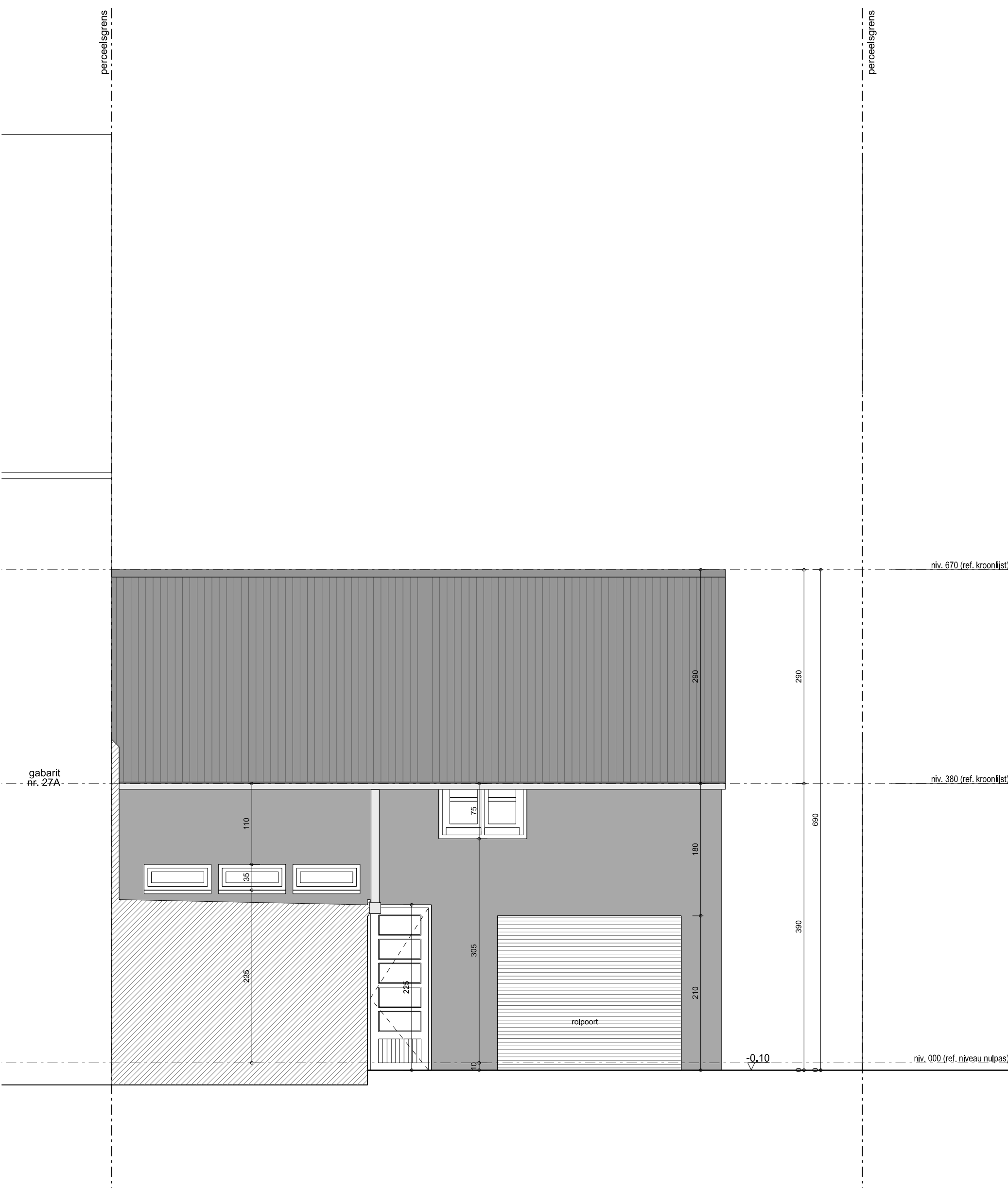
Gevelaanzicht E
