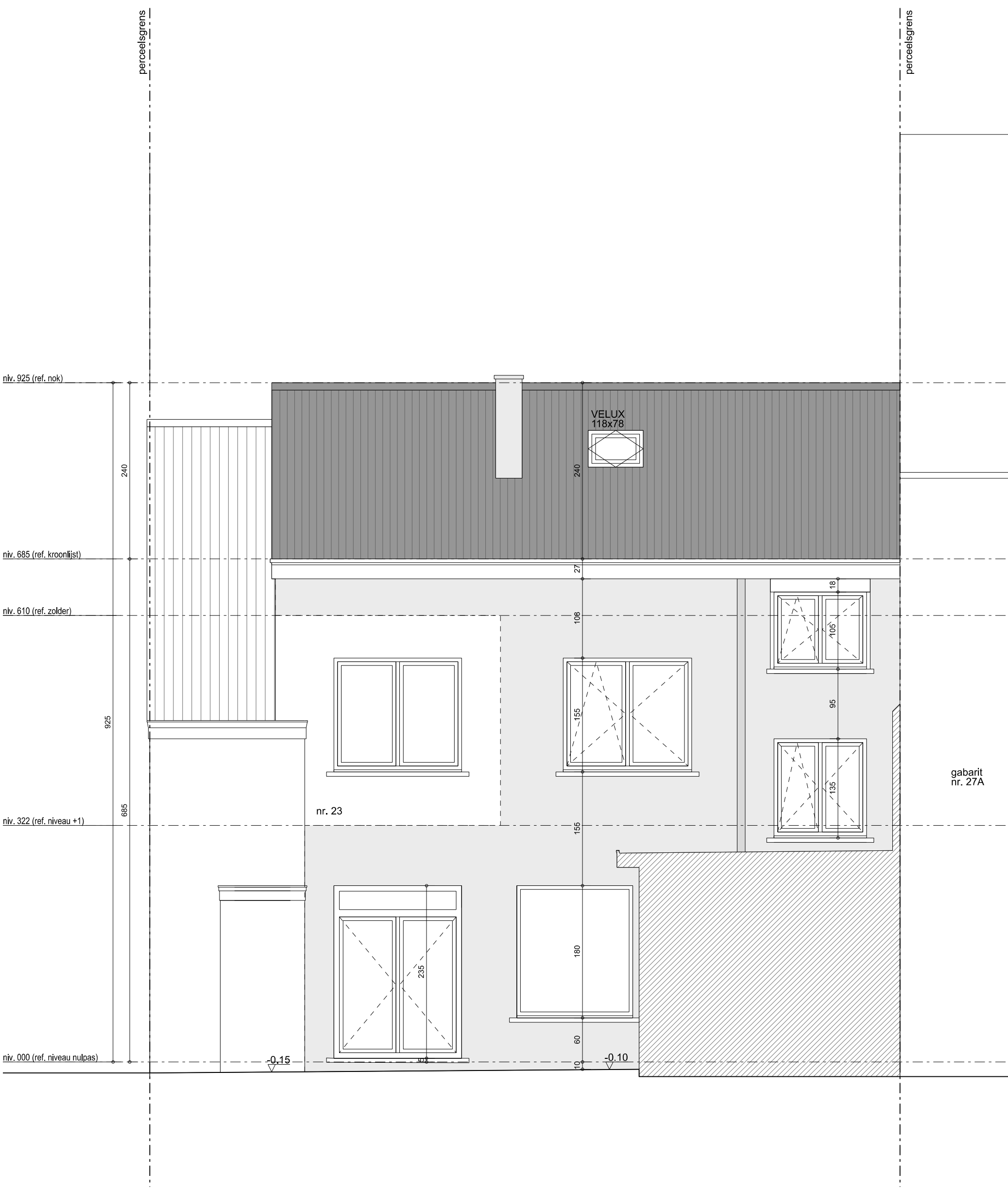
Gevelaanzicht D
