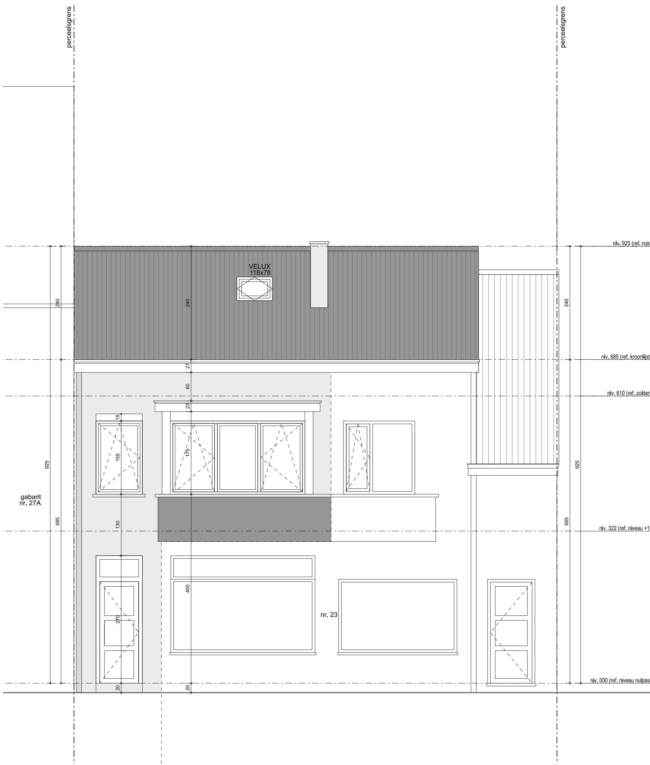
Gevelaanzicht A
