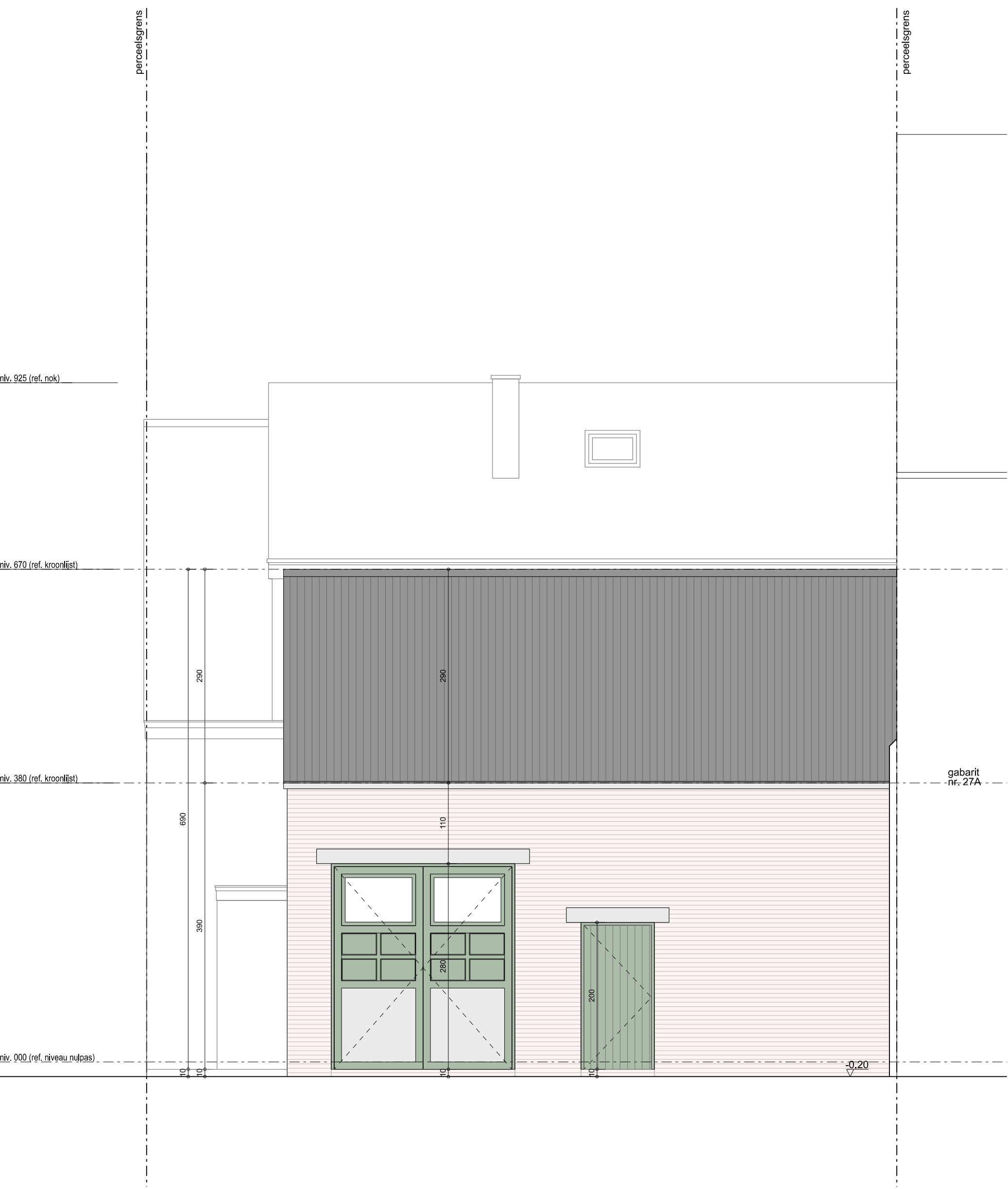
Gevelaanzicht C
